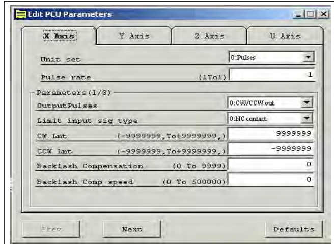
Configuración parámetros PCU
