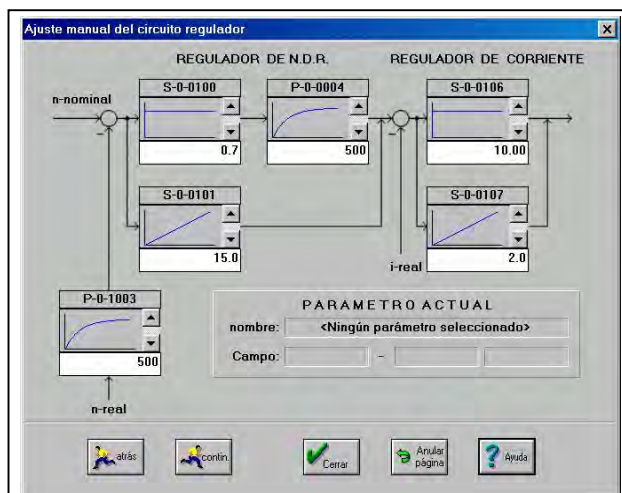
Ajuste manual del circuito regulador
