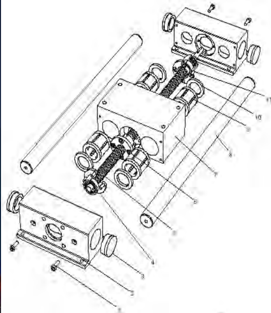
Despiece de husillo a bolas
