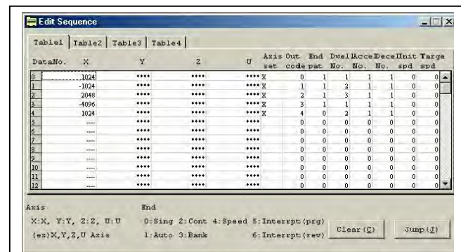
Configuración de secuencias predeterminadas
