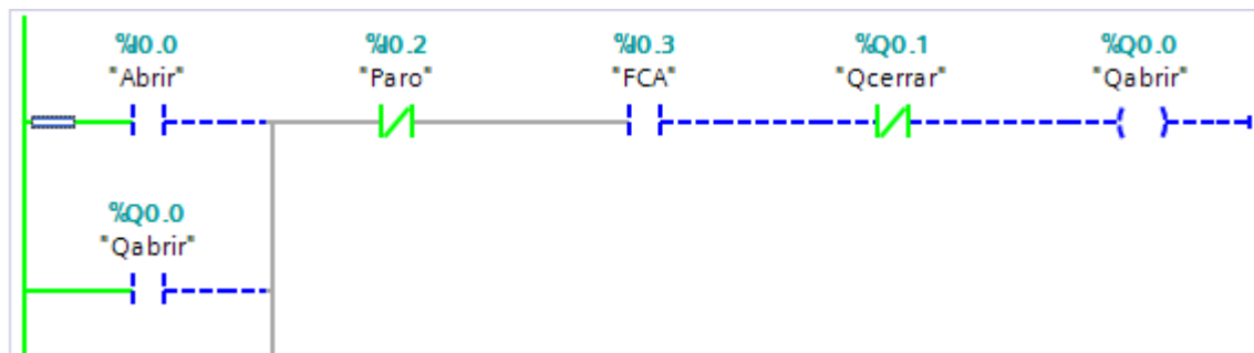
Figura 29. Observación del funcionamiento del programa.
