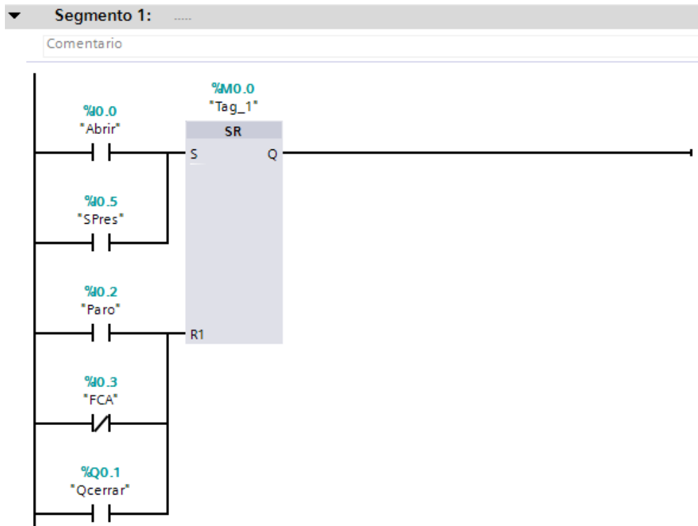
Figura 34a. Programa modificado con temporizadores y contador. Segmento 1
