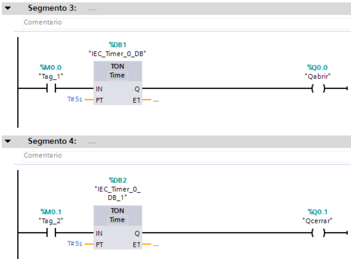
Figura 34c. Programa modificado con temporizadores y contador. Segmentos 3 y 4
