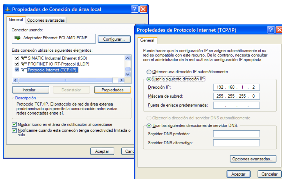
Figura 24. Dirección IP y máscara de subred de la PC.
