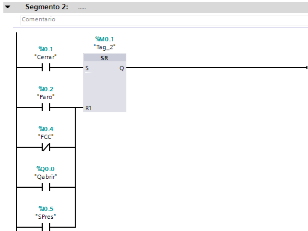
Figura 34b. Programa modificado con temporizadores y contador. Segmento 2
