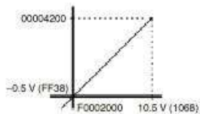
Eje horizontal: tensión de entrada, Eje vertical: dato BCD
