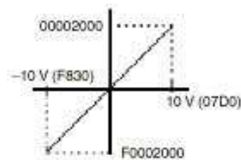
Eje horizontal: tensión de entrada, Eje vertical: dato BCD
